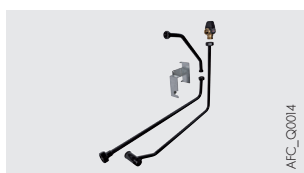
Kit hidráulico limitador de temperatura para circuito de suelo radiante en modo directo - Bulto MV10
