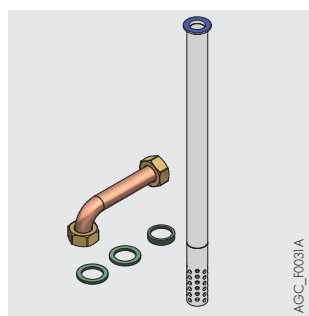
Kit de recirculación para el acumulador 100 HL - Bulto ER 218
