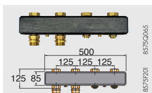
Colector para 2 ó 3 circuitos - Bulto EA140
